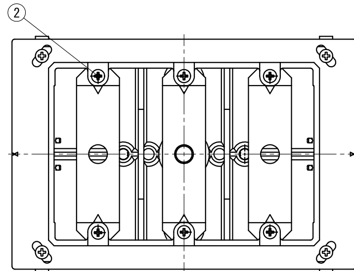
取付状態参考図 ( 1 / 2 )
